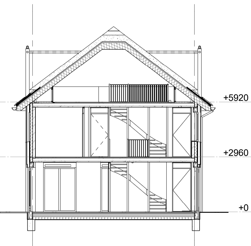
Blok E Doorsnede A-A 1 : 100
