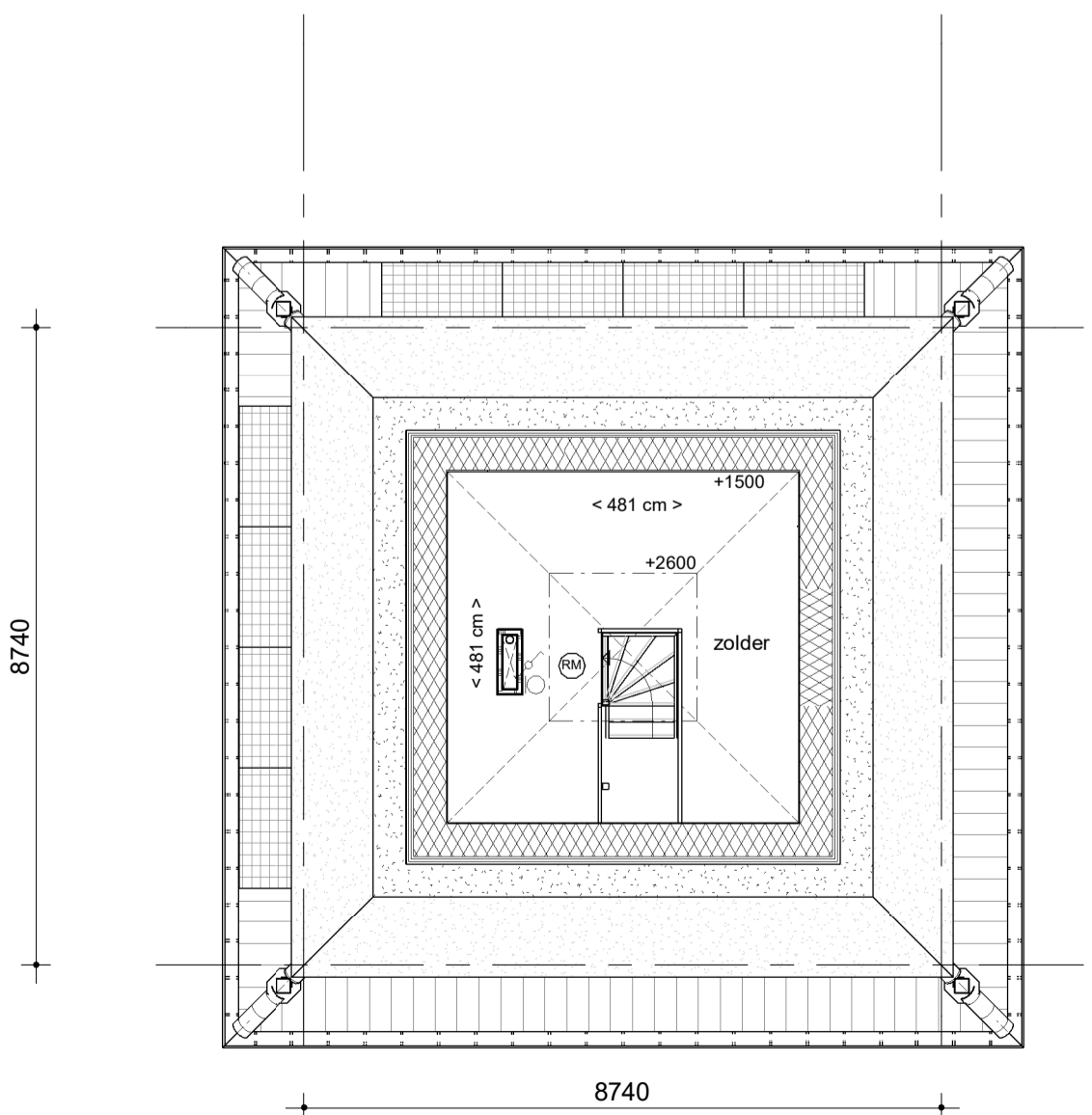
Blok E tweede verdieping type E 1 : 100 bnr. 24
