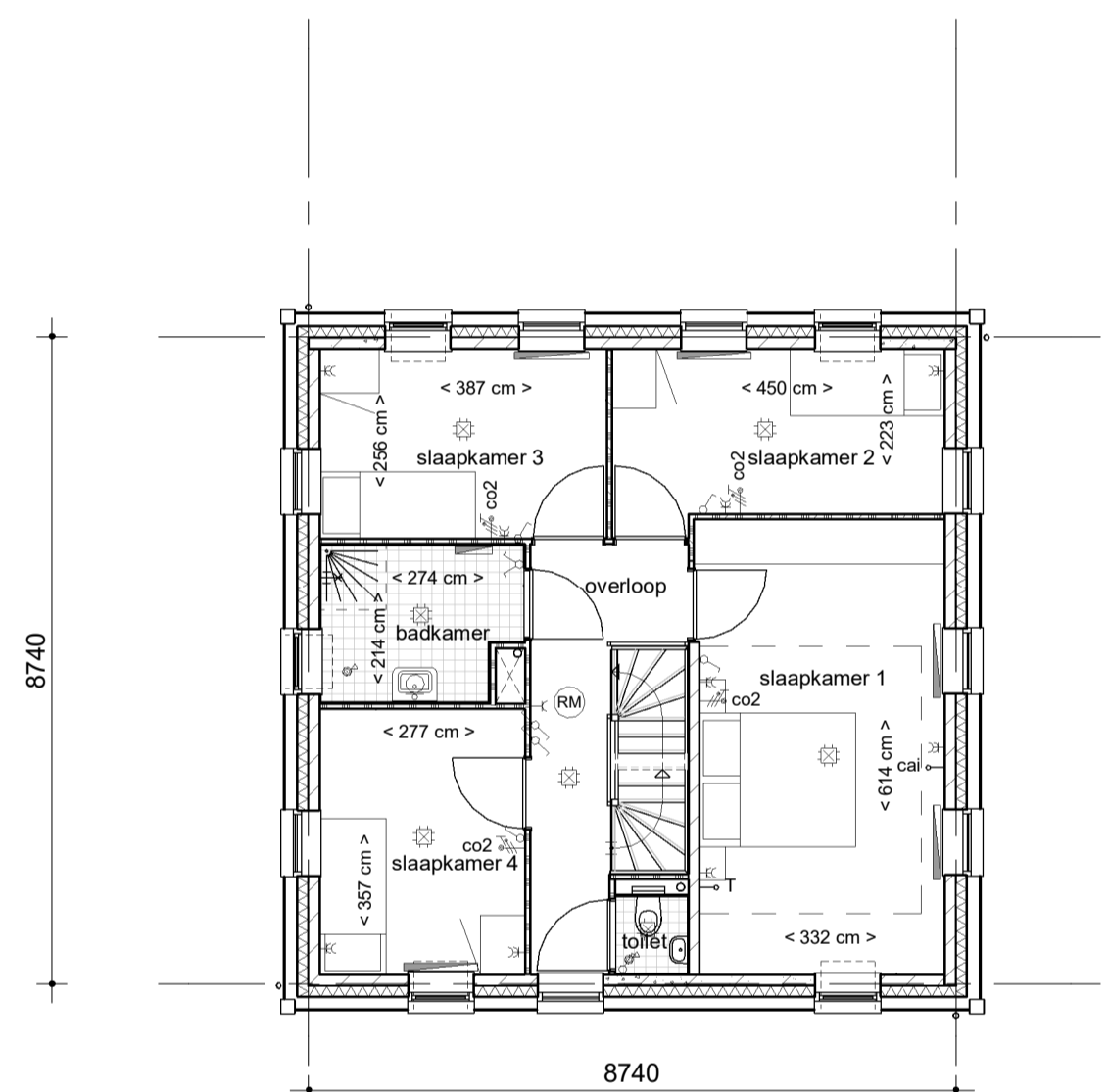
Blok E eerste verdieping type E 1 : 100 bnr. 24
