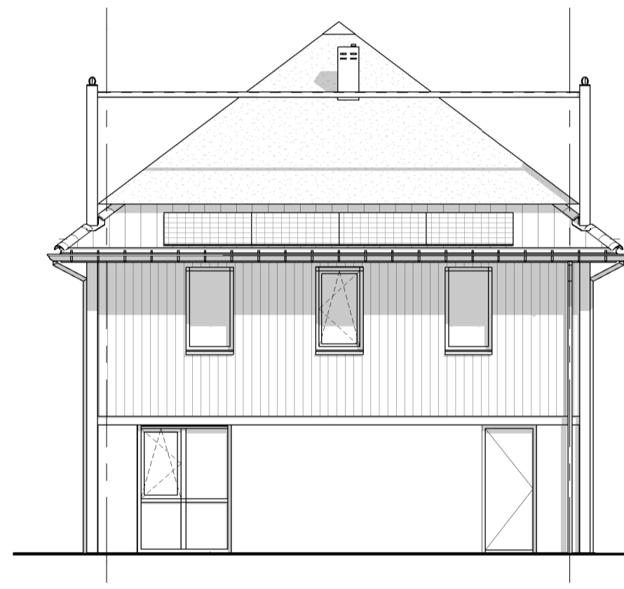
Blok E linkergevel type E 1 : 100 bnr. 24
