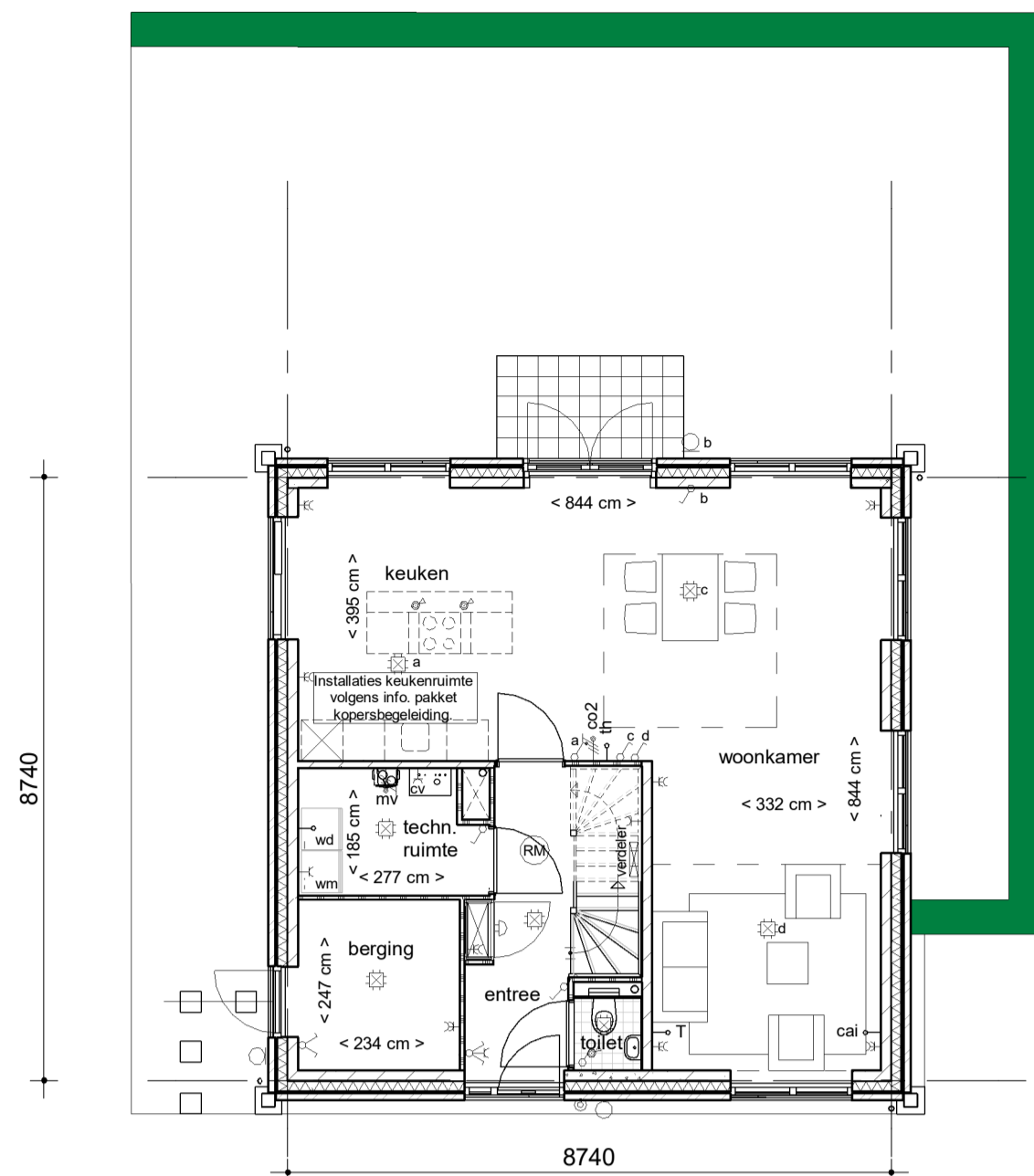
Blok E begane grond type E 1 : 100 bnr. 24
