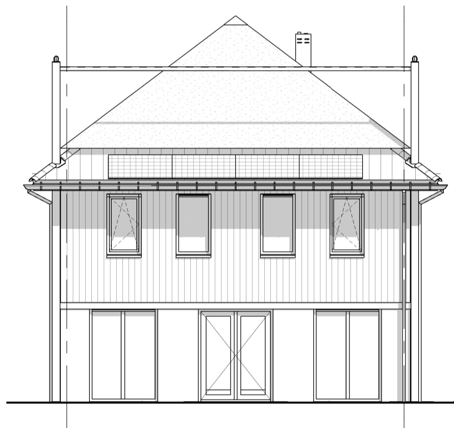
Blok E achtergevel type E 1 : 100 bnr. 24
